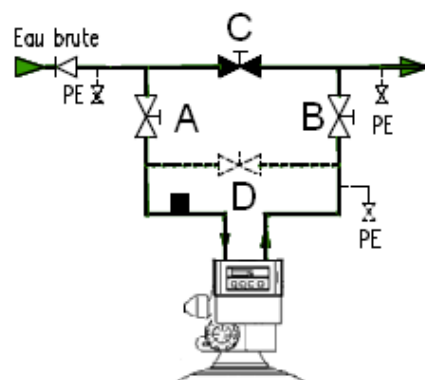
Schéma n° IX - " Repérage vannes "
