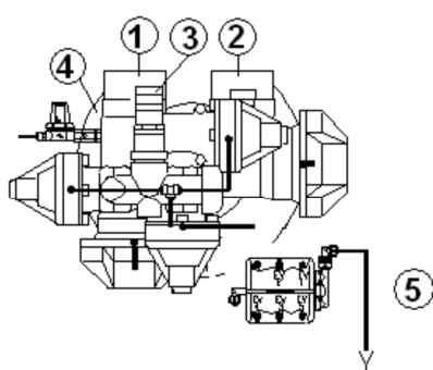
Schéma n° VIII - " Raccordements hydrauliques type 9000"
