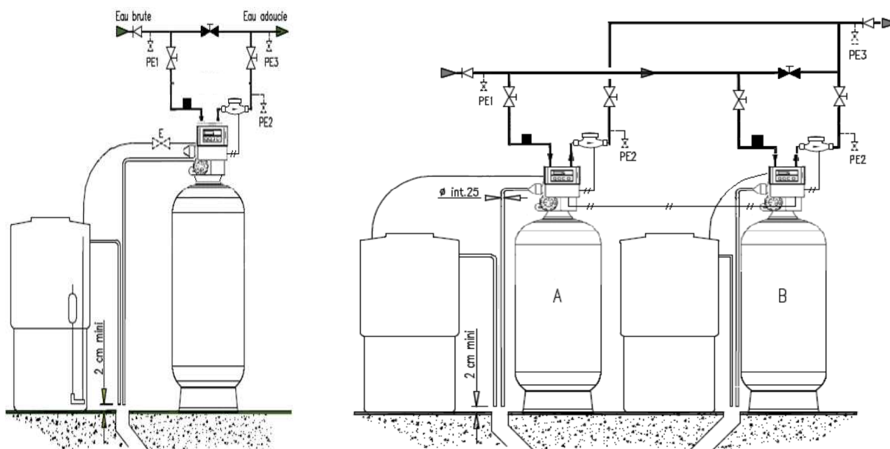
Schéma n° IV - " Adoucisseur simple à régénération sur base volume "
