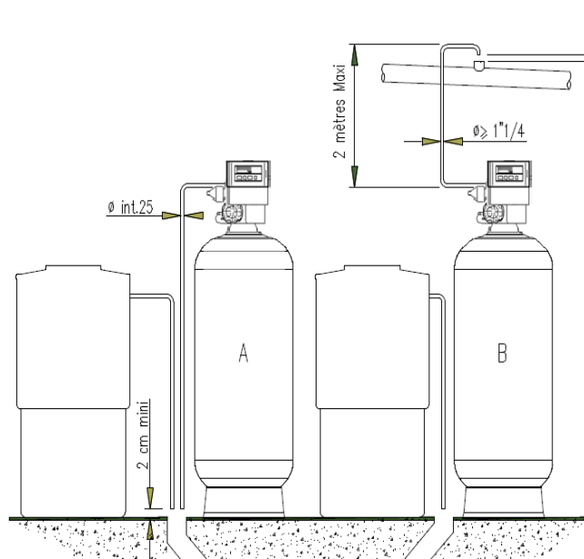
Schéma n° X - " Rupture de charge "
