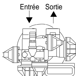
Montage sans bippasse
