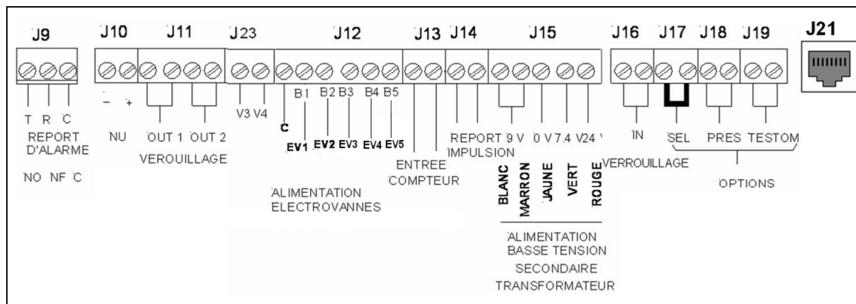
Schéma n° XIII - " Bornier de raccordements "
