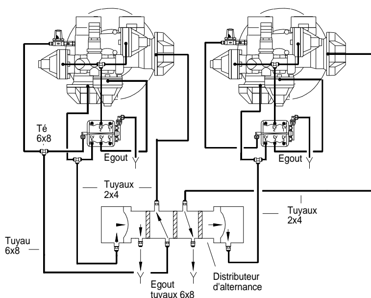
Schéma n° XII - " Raccordements hydrauliques d'alternance pour le type 9000"
