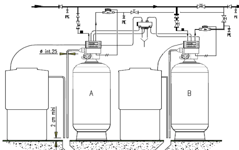
Schéma n° VI - " Adoucisseurs duplex au volume en alternance, 2 compteurs émetteurs "
