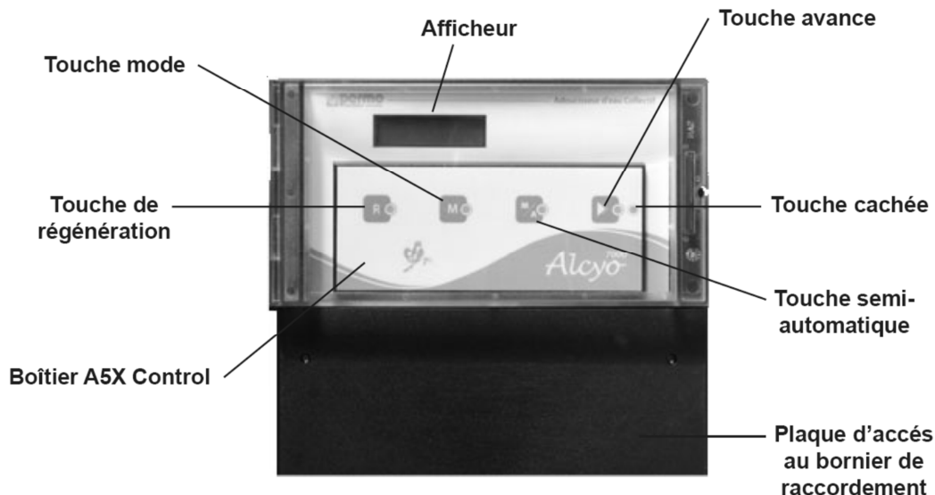
Schéma n° XVII - " Description du coffret "
