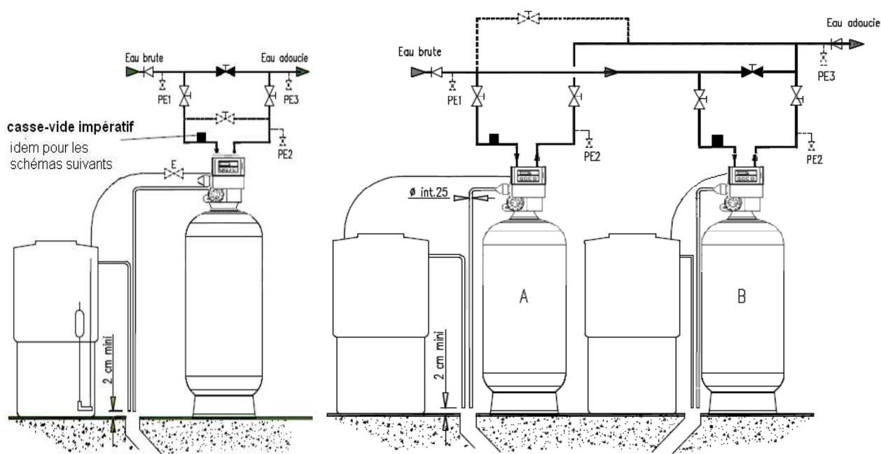
Schéma n° II - " Adoucisseur simple à régénération sur base temps "
