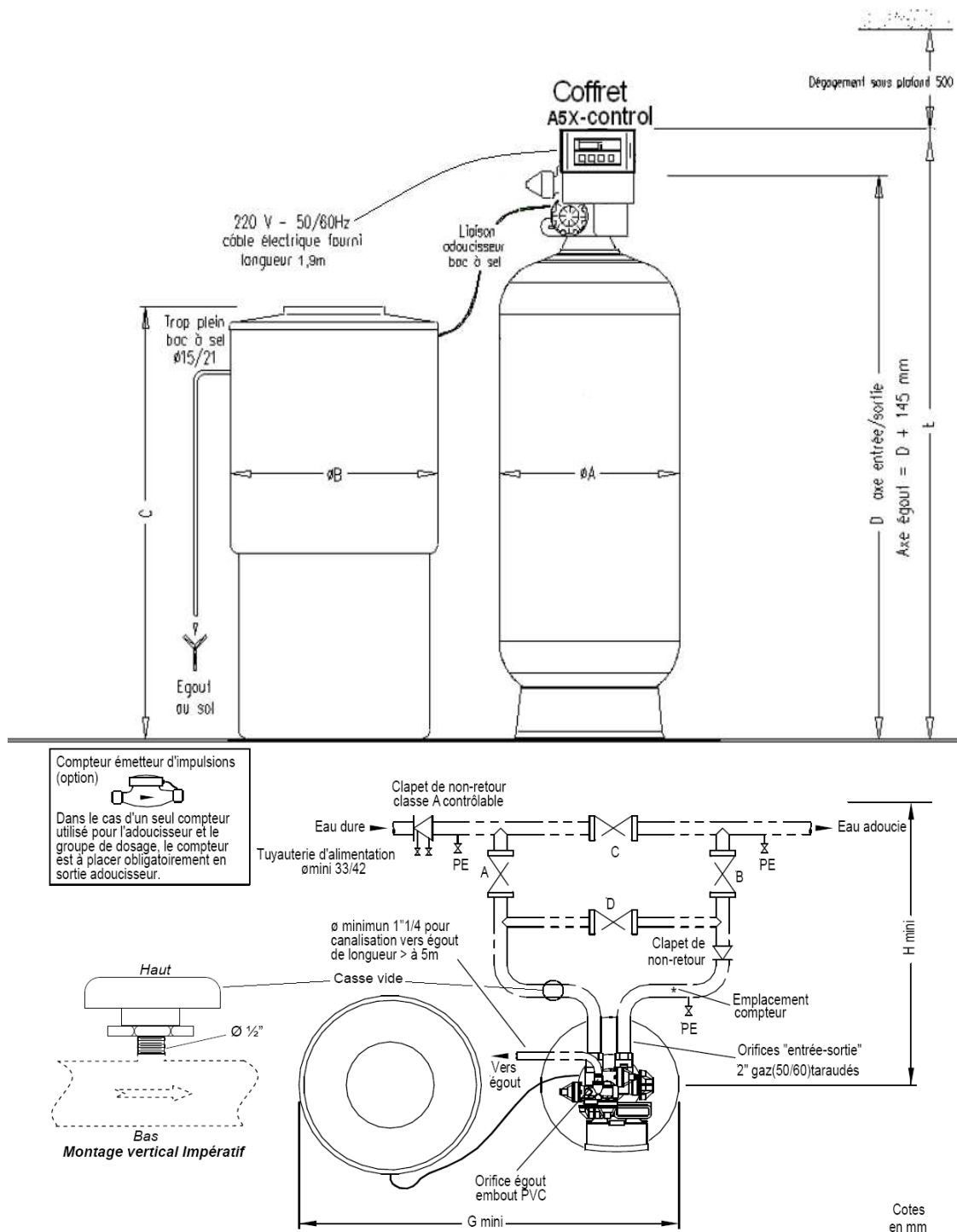
Schéma n° I - " Encombrement "
