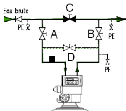
Schéma n° XIX " Repérage des vannes
