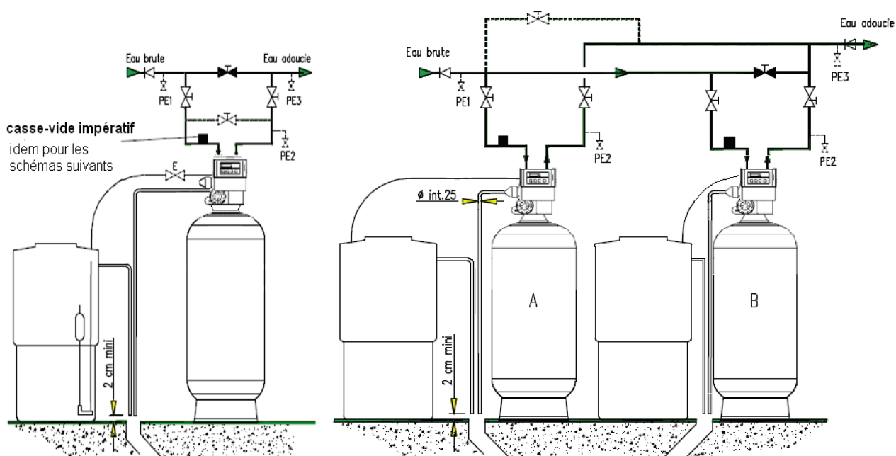
Schéma n° II - " Adoucisseur simple à régénération sur base temps "
