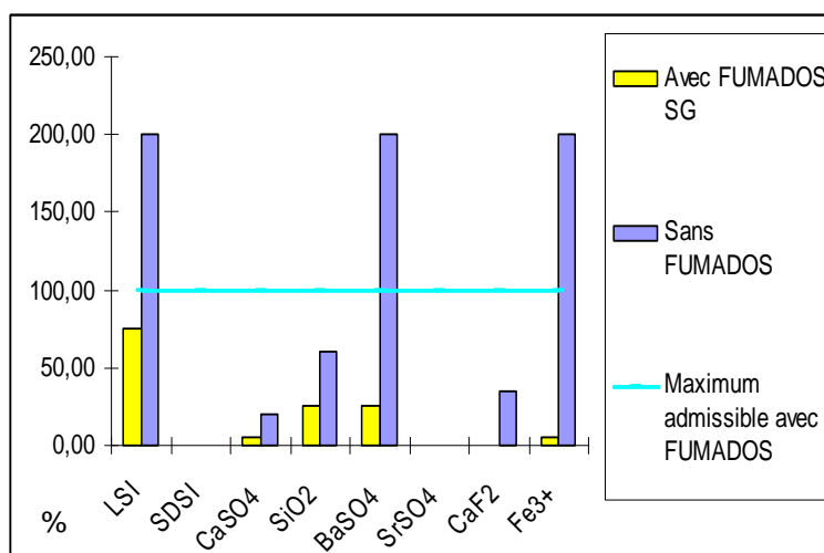
Figure 1 : Pourcentage de saturation dans le concentrat (exemple)
