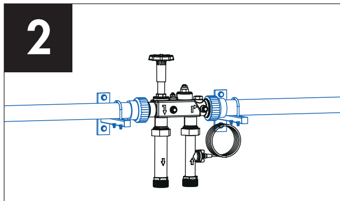
Mise en place du module de raccordement S.C.
