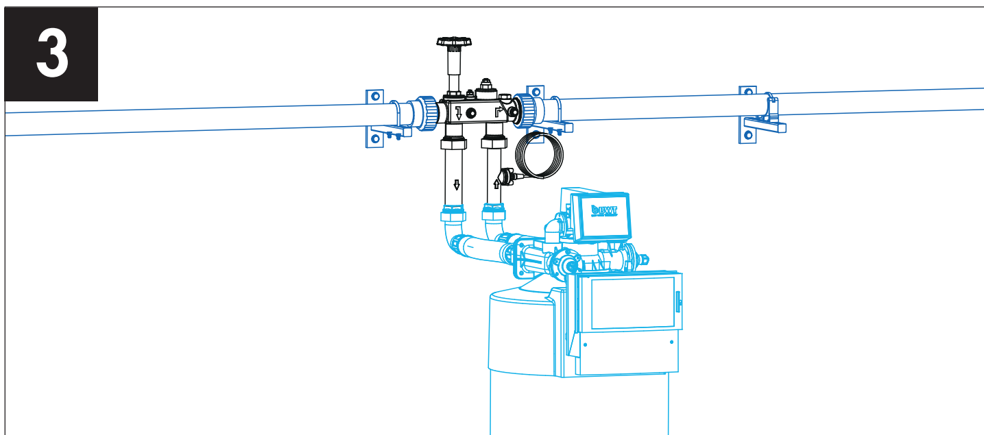
Raccordement de l'adoucisseur simplyconnect et mise en service.
