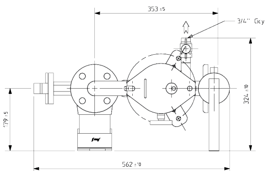
DESLUDGING UNIT 5/9
